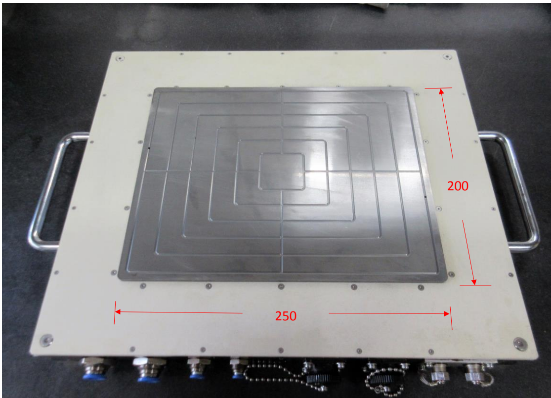
本体外形寸法 (取手部、配管継手除く) 355 x 380 x 48 (mm)
